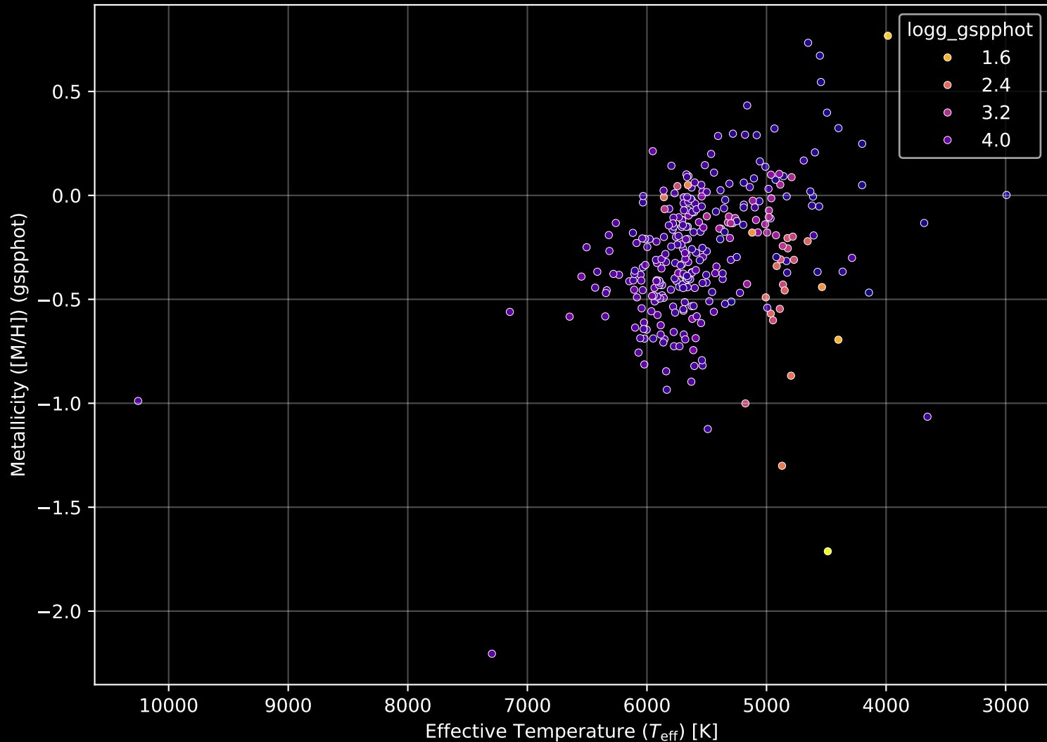
GALAH DR4 Field: [7045] Stellar Population Parameters (n= 305)
